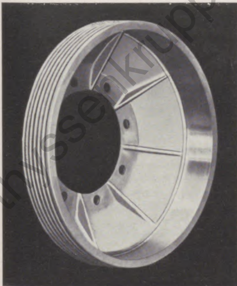
Bremstrommel mit Kühlrippen
