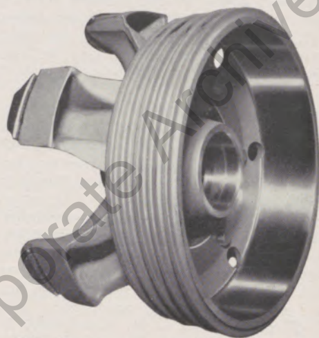
Trilix-Radstern mit montierter Bremstrommel
