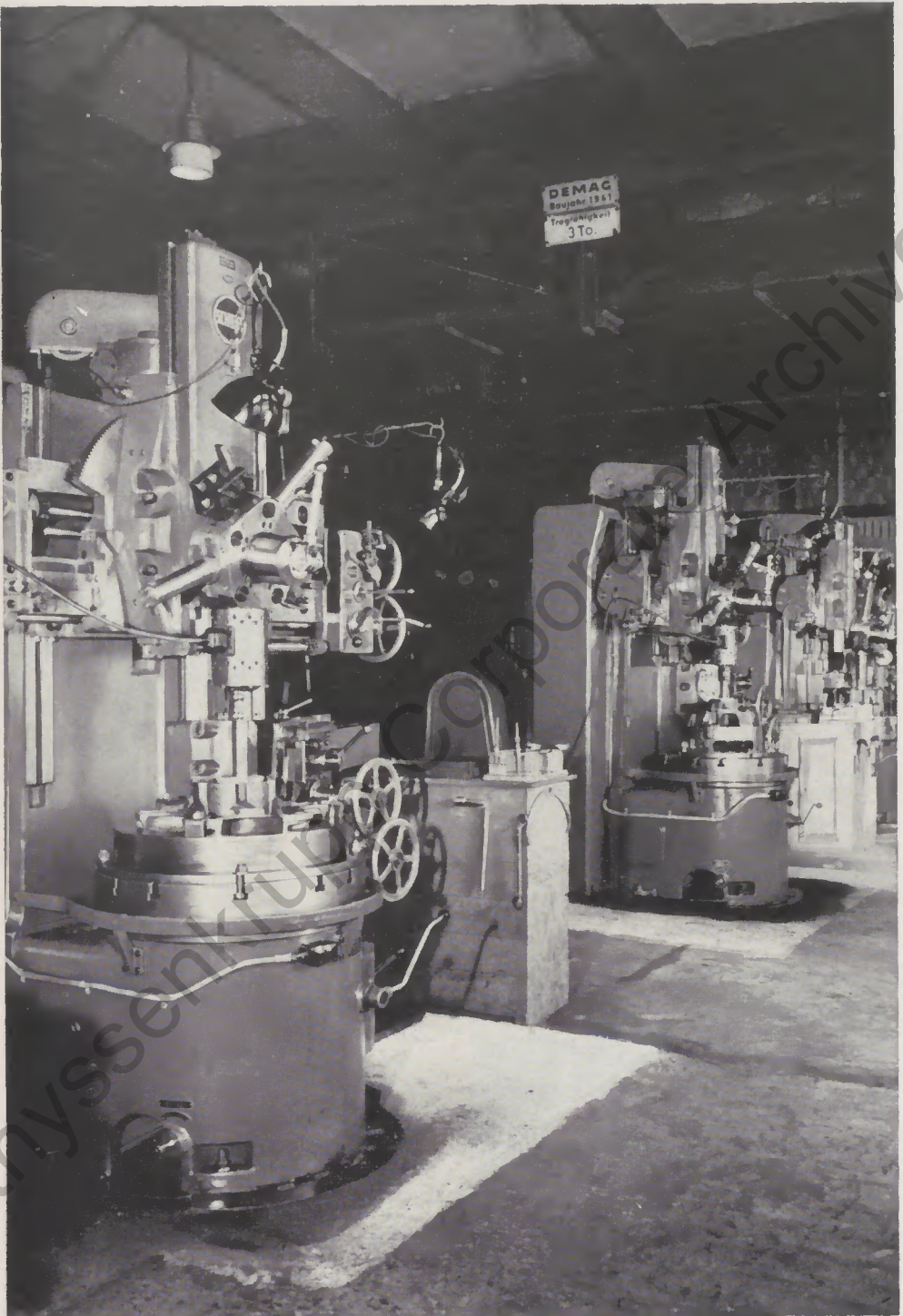
Vier neue Karusselldrehbänke im Bökerbau, Saal 2
