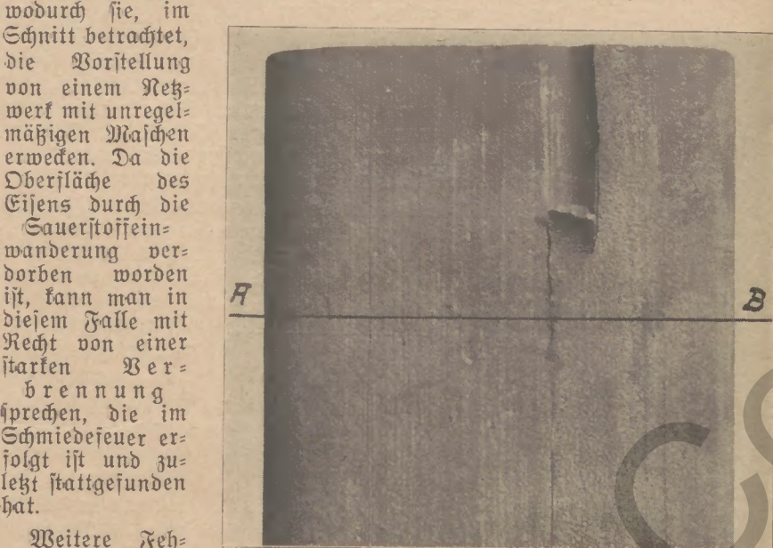
Abb. 11: Schienenlauffläche mit Absplittterung
