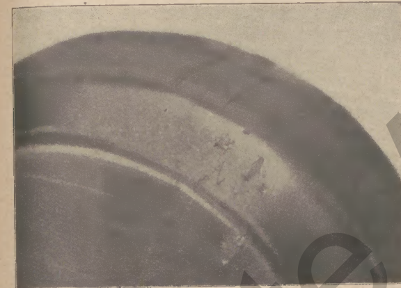
Abb. 4: Unterseite eines Blechnapfes; Abgüsse von der Haut, verursacht durch darunterliegende kleine Schlackeneinschlüsse
