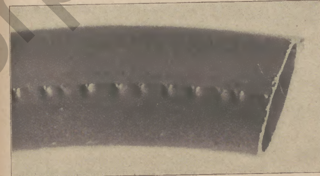
Abb. 5: Durch Schlackeneinschlüsse verursachte Aufsplitterung an einem Rohrmantel
