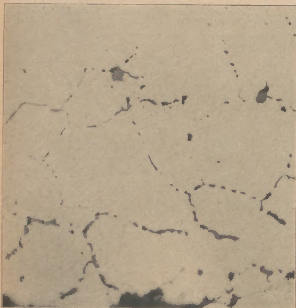
Abb. 10: Auf das Fünfhundertfache vergrößerter Schnitt durch die in Abb. 9 dargestellten Oberflächenaufrauungen; große Verbrennungsercheinungen. Die Schlacken sind Eisenzunder
