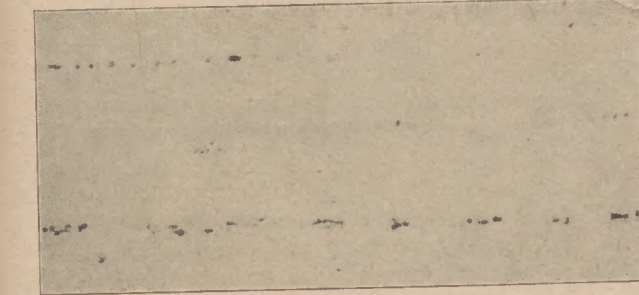
Abb. 6: Hundertsach vergrößerter Längsschnitt durch einen schlechten Automatenstahl; an den harten, dunklen Schlackeförnchen hat sich der Drehmeißel rasch stumpfgerieben
