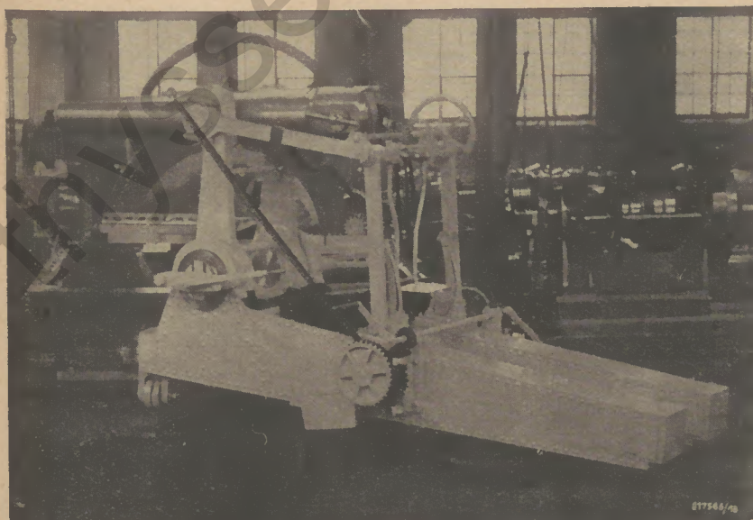
Interessante Geschützkonstruktion aus der „Gussstahl- und Waffen-Fabrik Witten vorm. Berger & Comp.“
