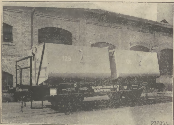
Bild 16: Zweiaxiger Küberwagen zum Erztransport
