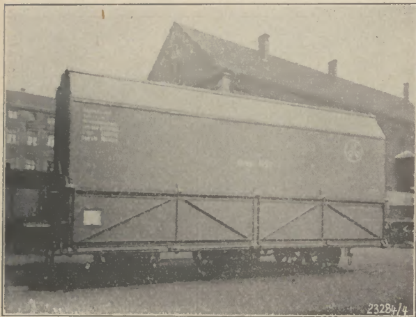
Bild 15: Dreiaxiger Großraum-Sattelwagen für die Dortmunder Union
