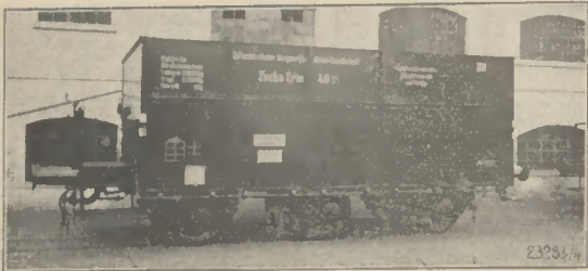
Bild 14: Zweiaxiger Sattelwagen, sogenannter Efselrückentwagen
