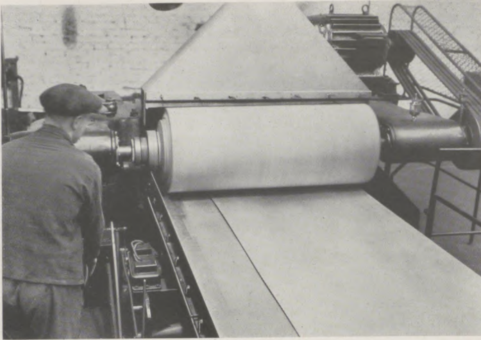
Abbildung 3: Flächenschleifmaschine
