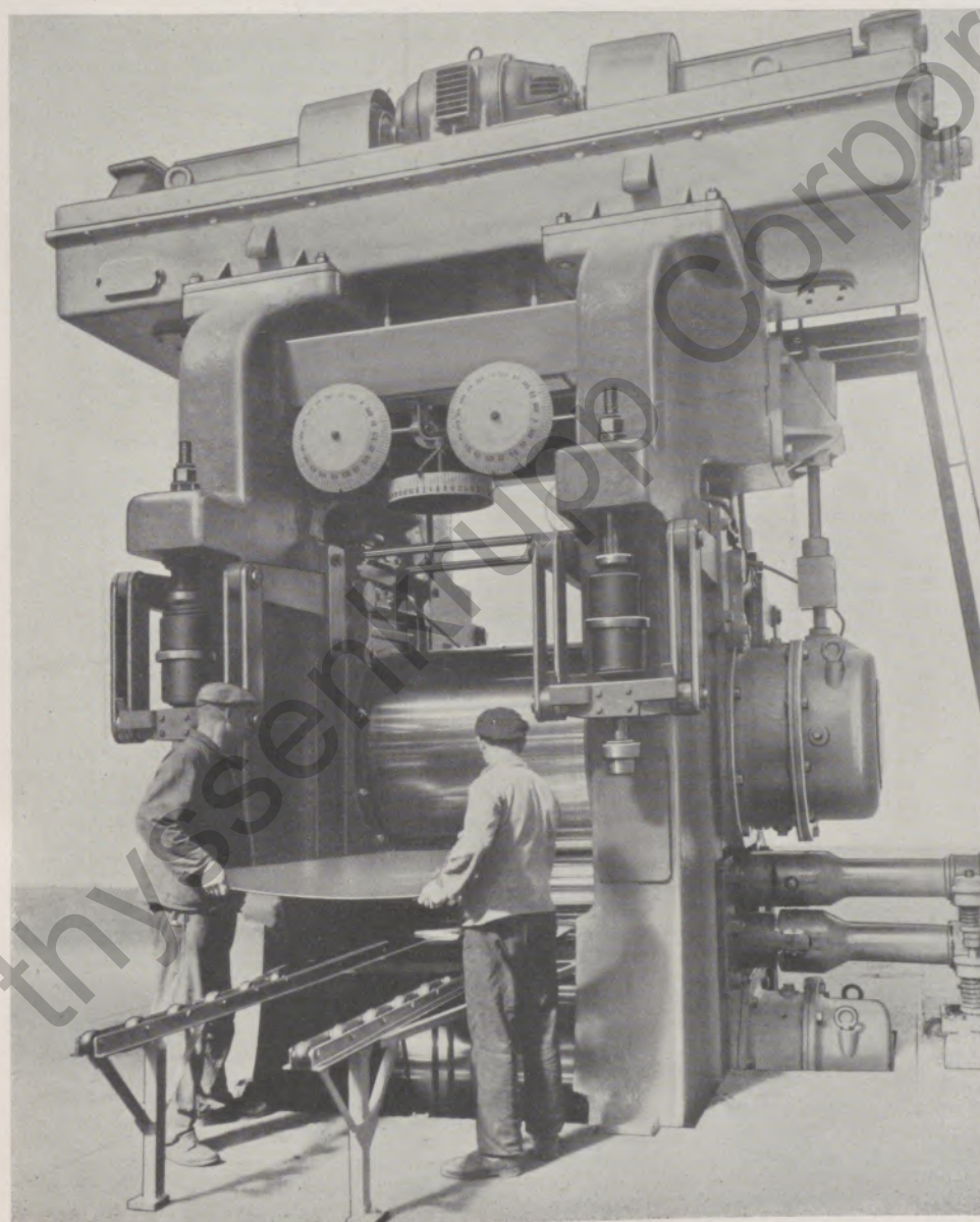
Abbildung 2: Kaltwalzengerüst
