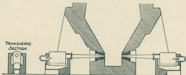
Die Windeinführung im ersten Neilsonschen Winderhitzer.
