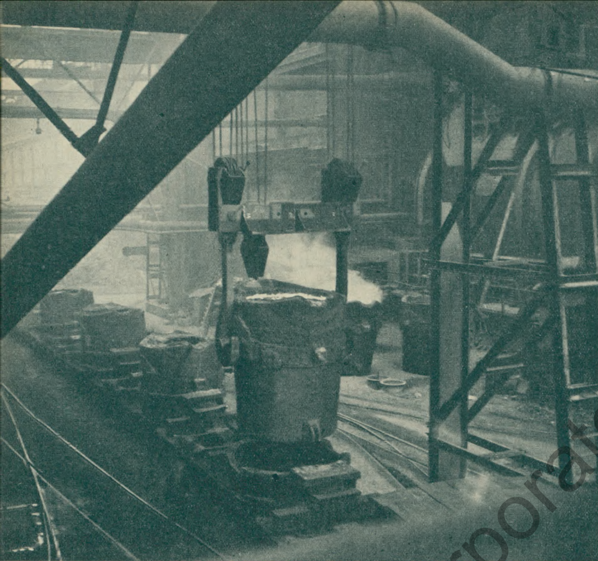
2. Die bis an den Rand mit flüssigem Eisen gefüllte Pfanne wandert zum Roheisenmischer, dessen Umriffe im Hintergrunde rechts sichtbar sind.
