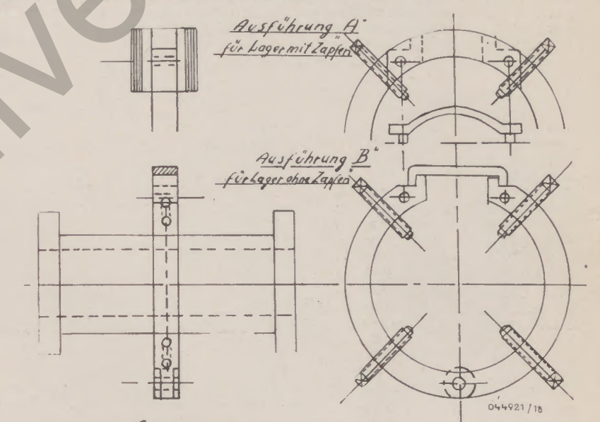
Spannring zum Drehen geteilter Lagerschalen.
