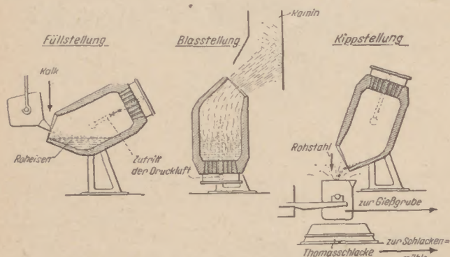
Schema einer Thomasbirne
