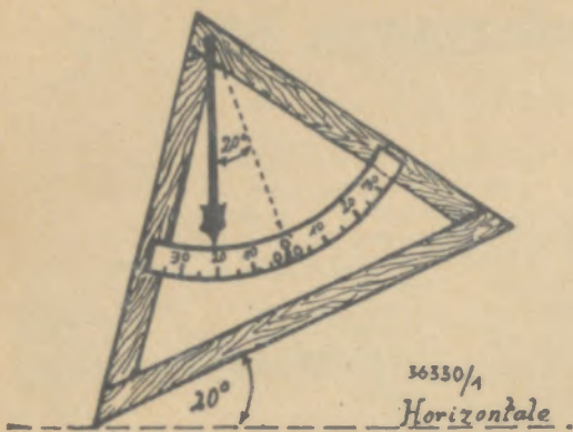
Fig. 10: Neigungsmesser
