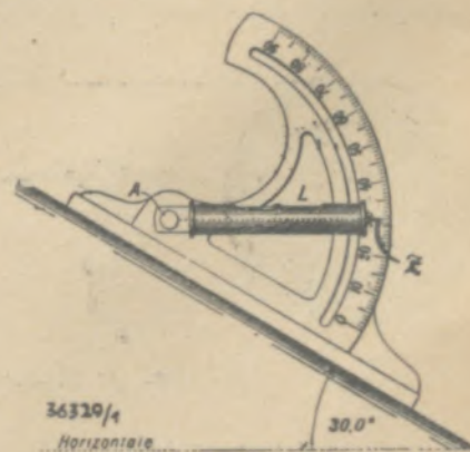
Fig. 9: Libellengradwaage
