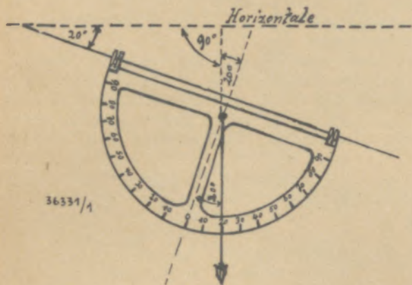
Fig. 11: Gradbogen
