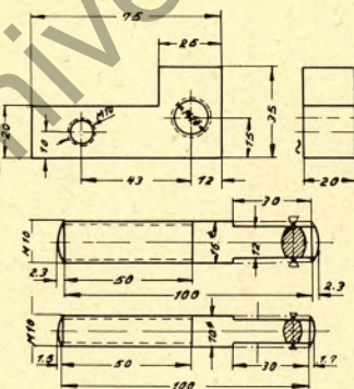
Winkelstück mit Schrauben
