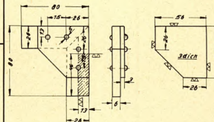
Genietete Eckverbindung
