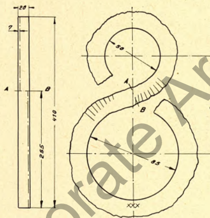
Gehämmerter Bandstahl
