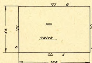
Rechteckplatte
