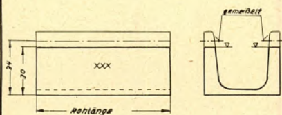
Abgefeilter U-Stahl
