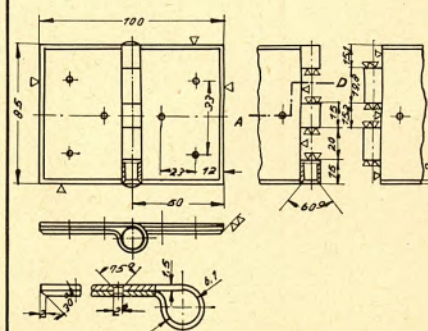
Gelenkband
