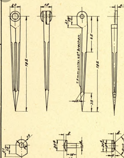
Spitzzirkel
