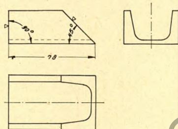
Abgeschrägter U-Stahl
