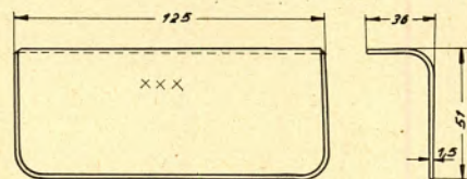
Blechbacke für Schraubstock
