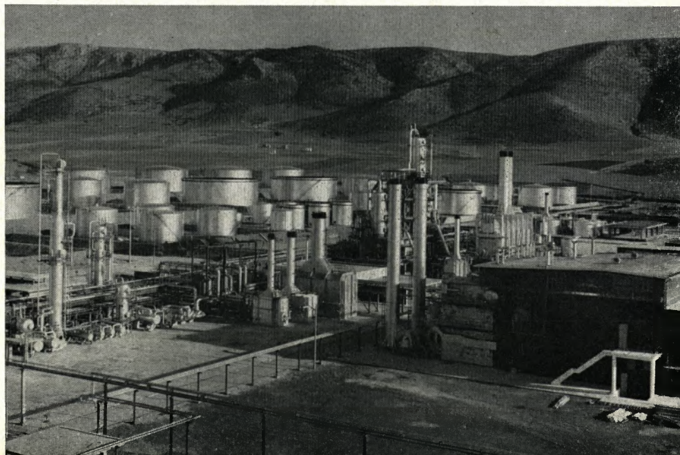
Am 5. November weihte König Paul von Griechenland die Ölraffinerie Aspropyrgos ein, die durch Krupp, Hydrocarbon Mineralöl und Stahlunion Export erbaut wurde. Die gesamte Rohrlieferung erfolgte durch Phoenix-Rheinrohr und die komplette Verrohrung durch unsere „Tochter“ Vereinigter Rohrleitungsbau
