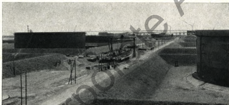
Mächtige Öltanks stehen am Beginn der Nord-West-Ölleitung in Wilhelmshaven. An ihrem Bau ist Phoenix-Rheinrohr beteiligt. Unser Unternehmen lieferte Grobbleche
