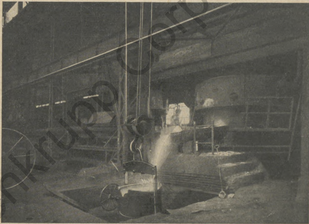
Abstich am Kupolofen
