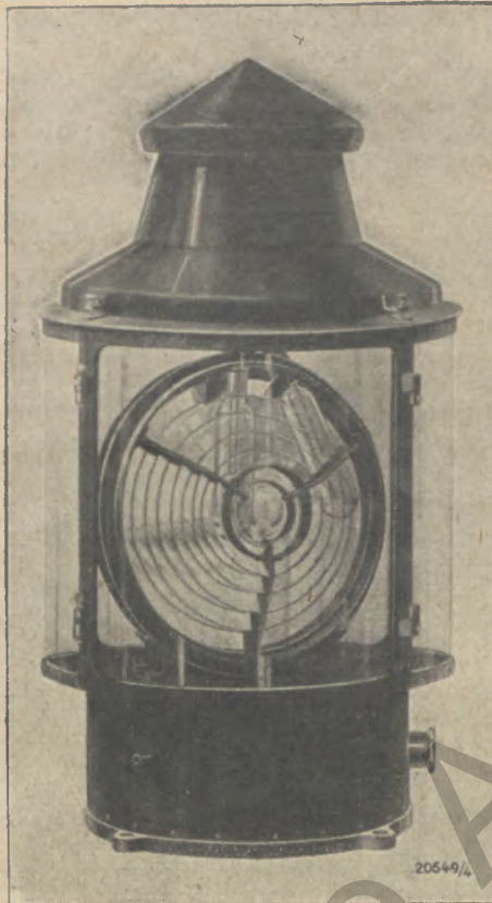
Drehlinseleuchte mit 300 000 Kerzen Lichtstärke
