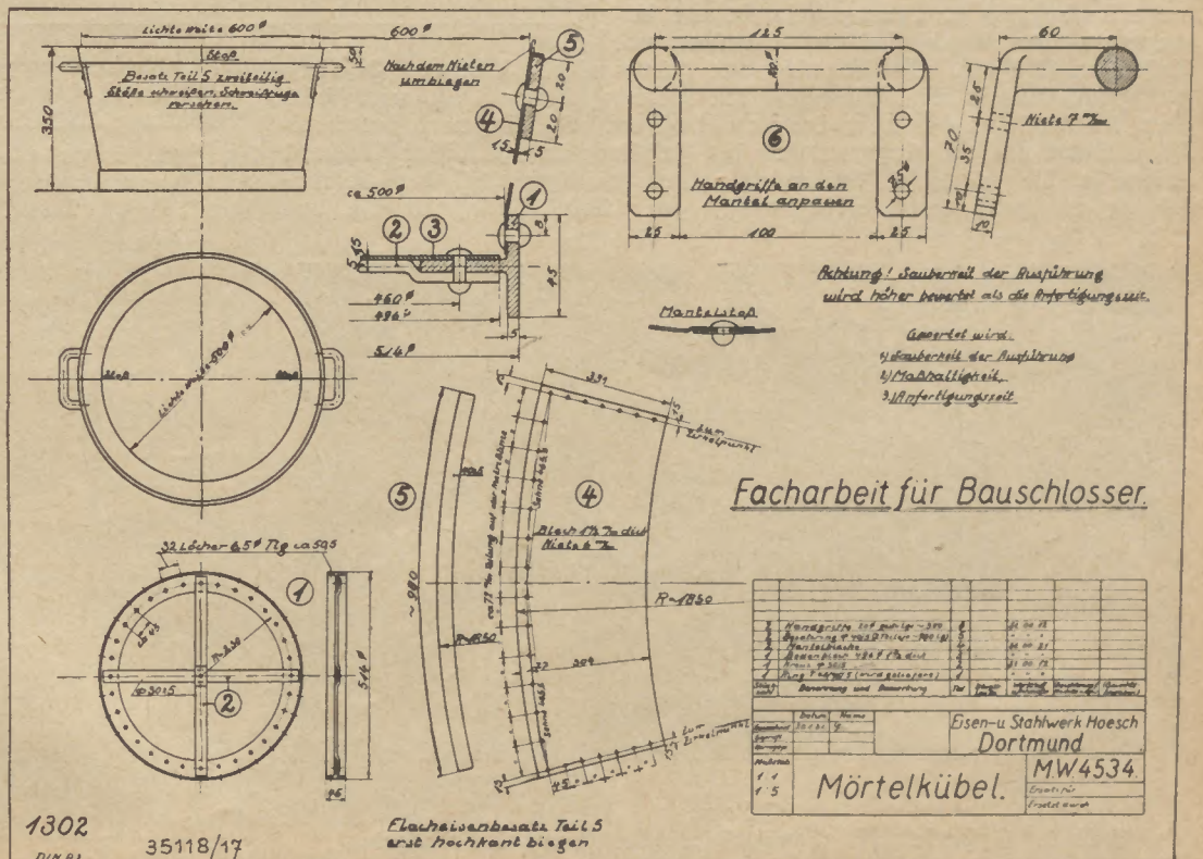
Bild 3: Facharbeit für Bauschlosser: Mörtelkubel, Aufgabe
