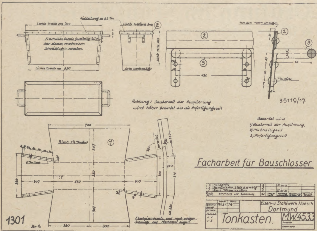
Oben: Bild 4: Facharbeit für Bauschlosser: Tonkasten, Aufgabe
