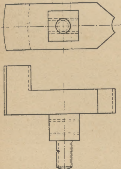
Zur Zeichenaufgabe I für Modellschreiner.
