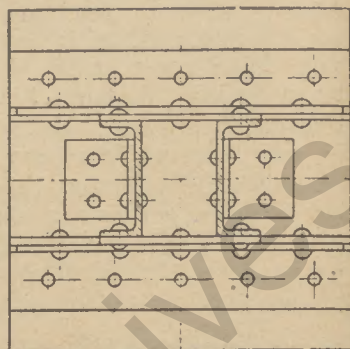
Draufsicht. Zeichenaufgabe für Bauschlossler.
