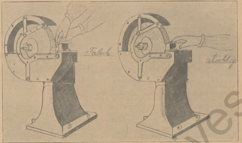
Falsche und richtige Stellung der Schleifvorlage an Schmirgelscheiben. Zeichnung von Betriebsführer a. D. Perlers.
