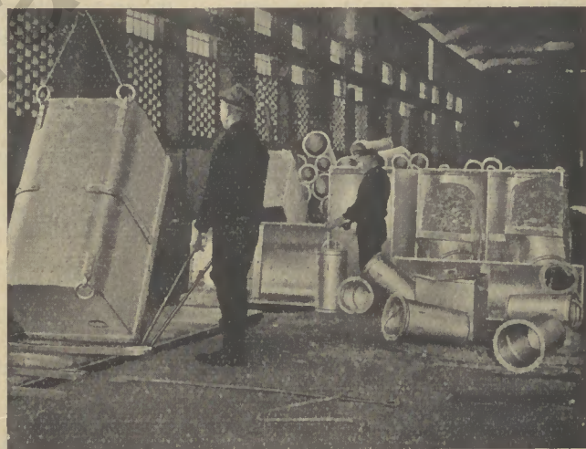
Bohrverzinkung eines kompletten Förderwagenkastens in unserer Ruhrstahl A.-G.
