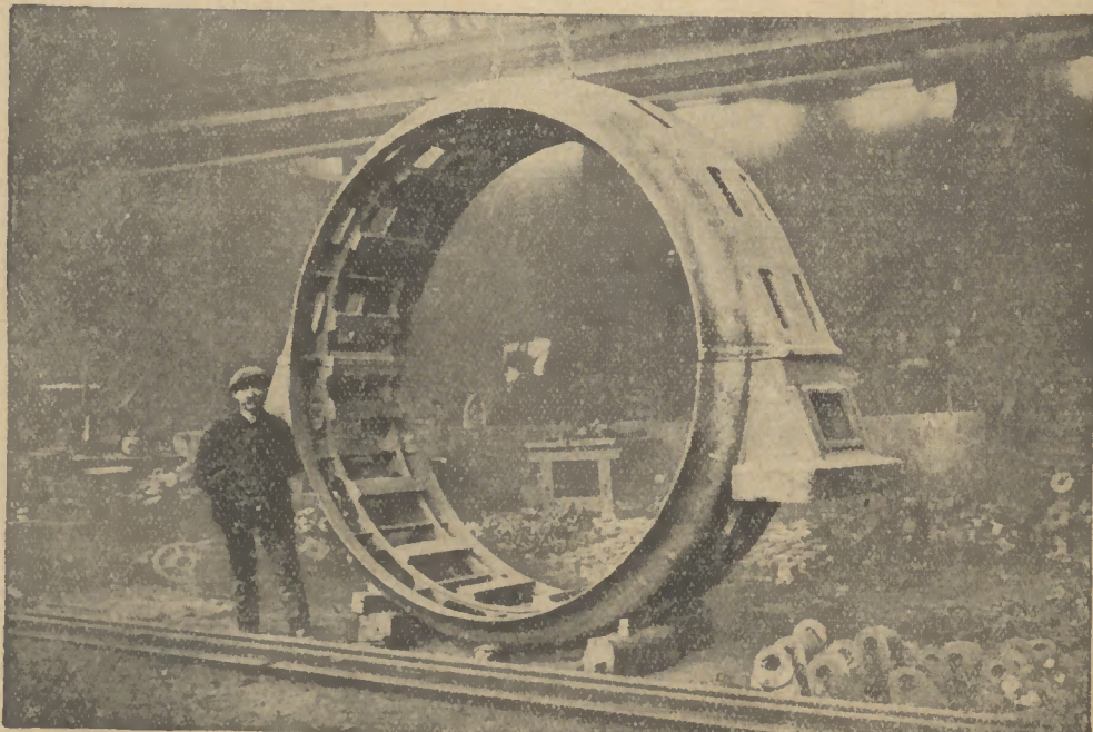
Motorgehäuse aus Eisenguß, zirka 4150 Kilogramm schwer
