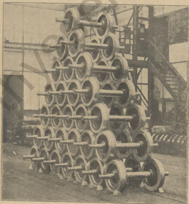
Schmalspur-Wagenradsätze für die serbischen Staatsbahnen
