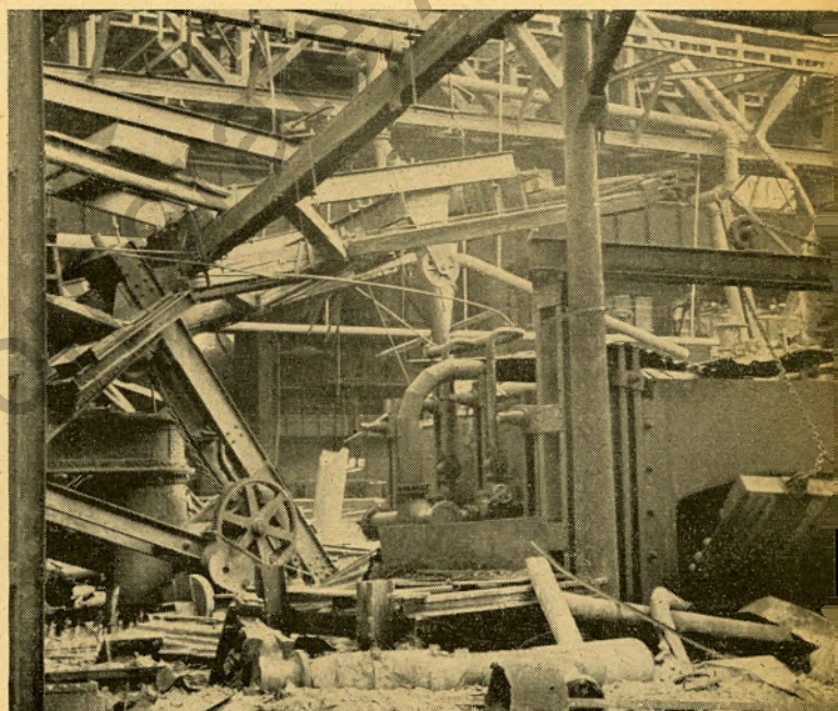
Hammerwerk
