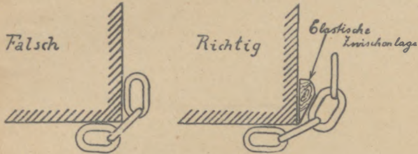
Schutz der Tragmittel beim Heben scharfkantiger Gegenstände durch weiche Zwischenlagen.
