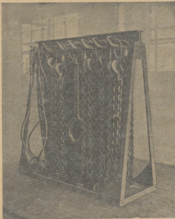
Die Aufbewahrung von Ketten und Seilen an Böden oder Gestellen.
