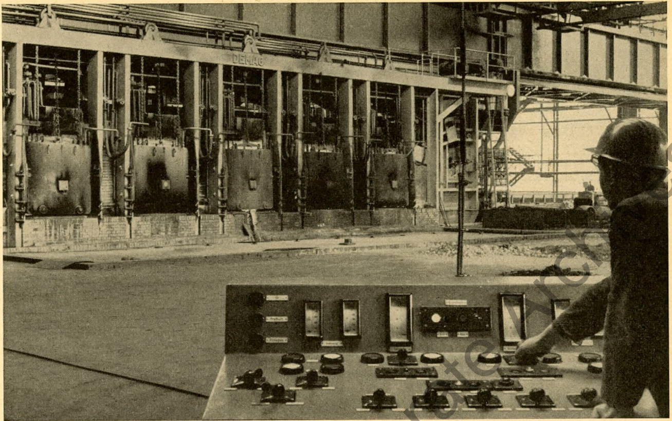
Vom Schaltpult aus überwacht und bedient der 1. Schmelzer seinen Ofen
