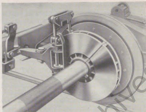
BSI-Scheibenbremse mit auf der Achse befestigter geteilter Scheibe
