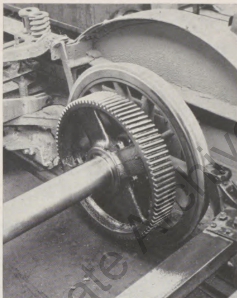
Zahnrad für Bahngetriebe
