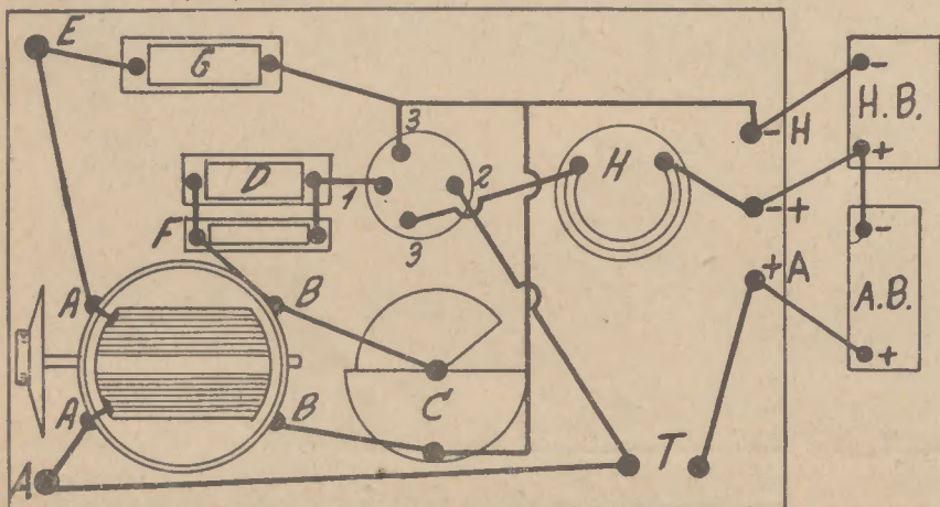
Abb. 1: Einröhrenrückkopplungsempfänger.
