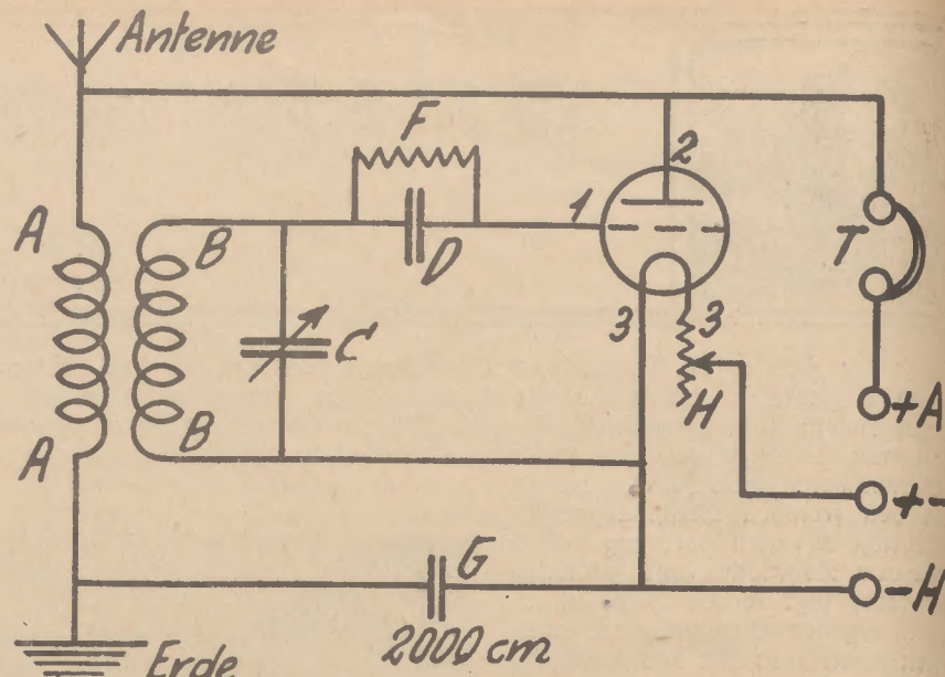
Abb. 2: Bauplan für den beschriebenen Empfänger.
