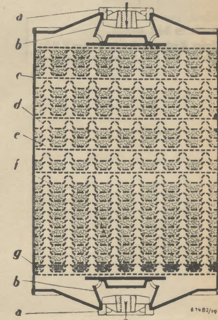
Abb. 12: Inneneinrichtung der Alkalipatrone
