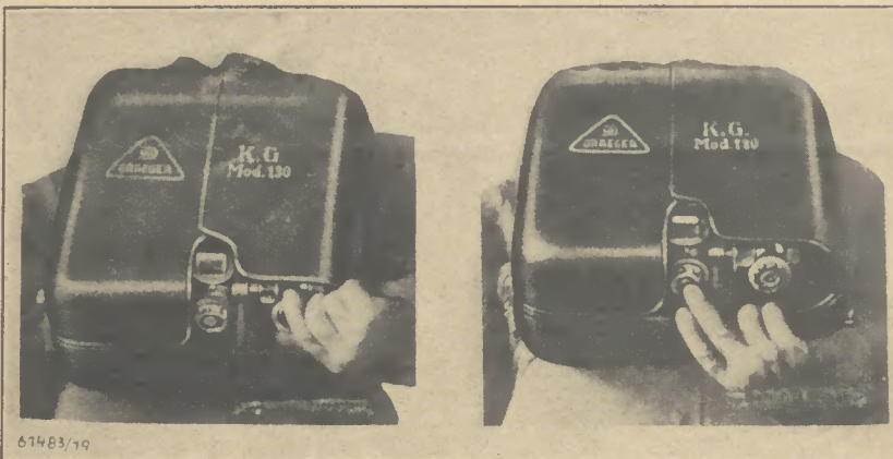
Abb. 13: Deffenen der Sauerstoff-Flasche (a) und Betätigung des Zusatzknopfes (b)
