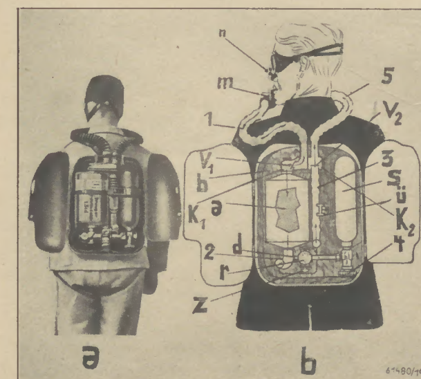
Abb. 10: Innenansicht und Aufbau des Sauerstoffgerätes
