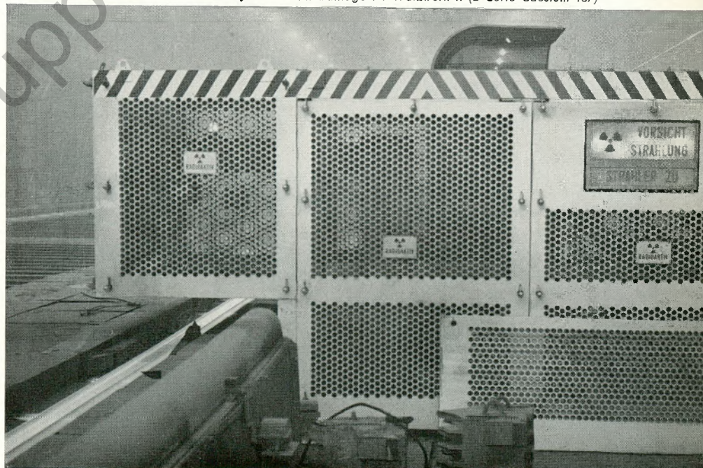
▼ Dickenmeßanlage im Walzwerk II (2 Curie Cäsium 137)
