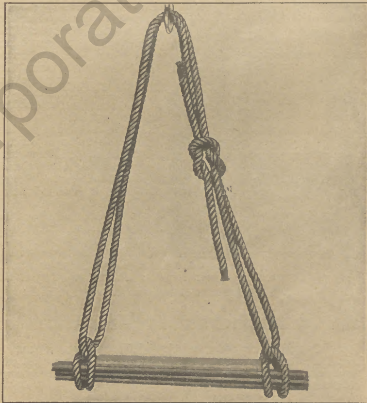
Doppelte Kreuzschlinge.
