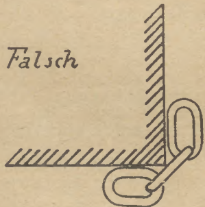
Schutz der Tragmittel beim Heben scharfkantiger Gegenstände durch weiche Zwischenlagen.
