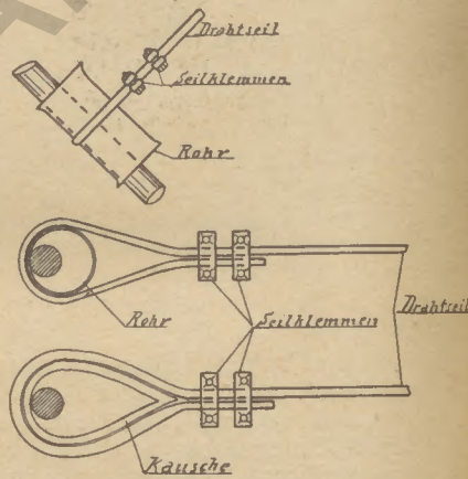
Herstellung von Schlaufen bei Drahtseilen mittels Seilklemmen.
