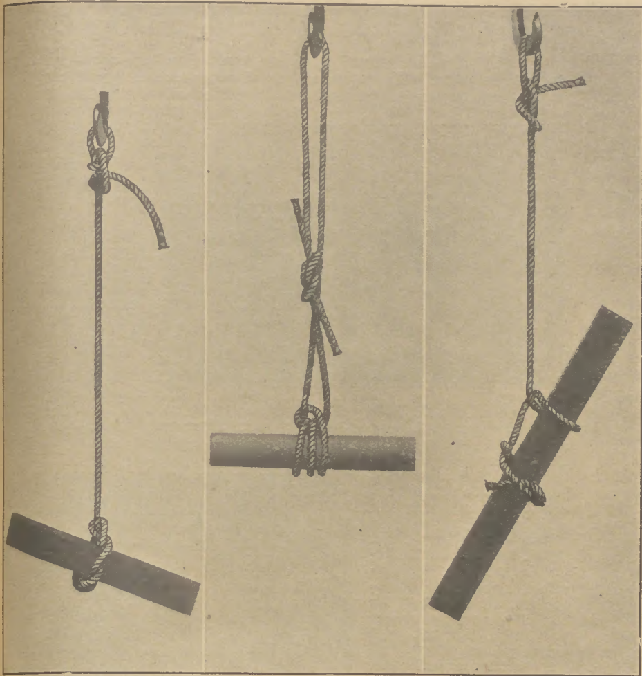
Zimmermannsknoten an der Last, Doppeltknoten am Haken für einfaches Seil (z. B. bei Transport unbelasteter Hölzer.)
