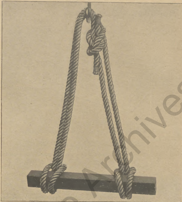
Doppelte Würgeschlinge.
