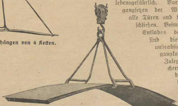
Transport von Platten mittels gekuppelter Traghaken.
