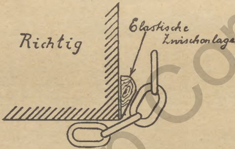
Schutz der Tragmittel beim Heben scharfkantiger Gegenstände durch weiche Zwischenlagen.
