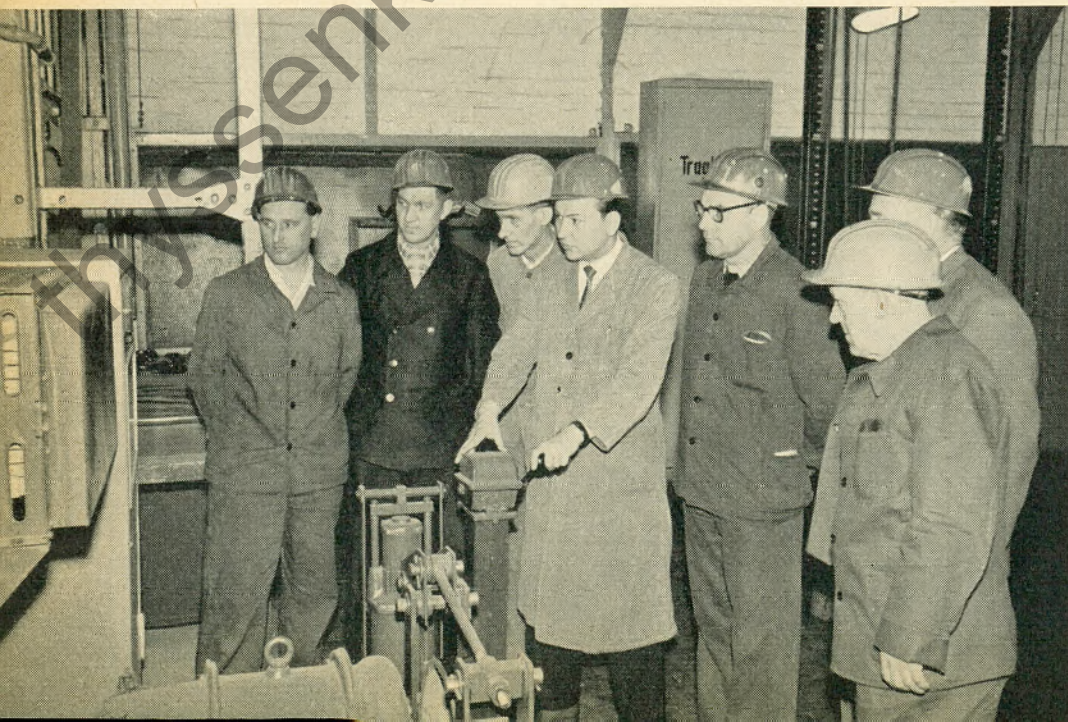
Hier werden die starken, bei plötzlichem Vor- und Rückwärtsschalten auf- tretenden Stromstöße abgelesen
