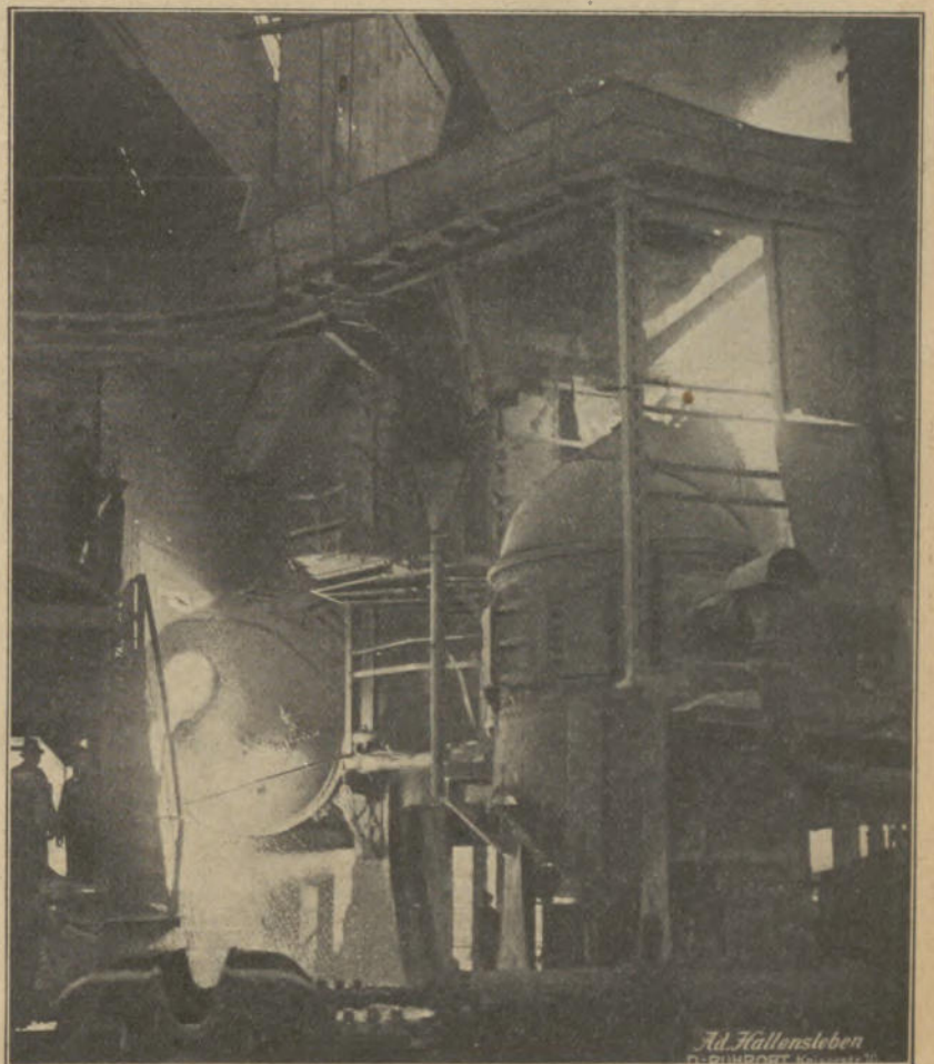
Rechts: Thomasbirne beim Blasen. Links: Abschütten der Thomaschlacke.
