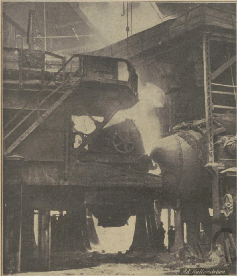
Zentralstrahl beim Einfippen des Roheisens.
