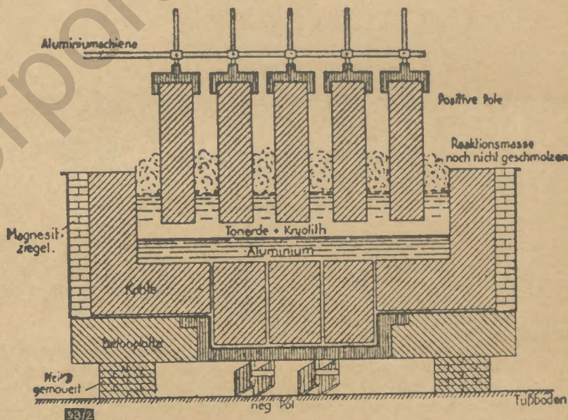
Schematische Darstellung eines modernen Aluminiumofens
