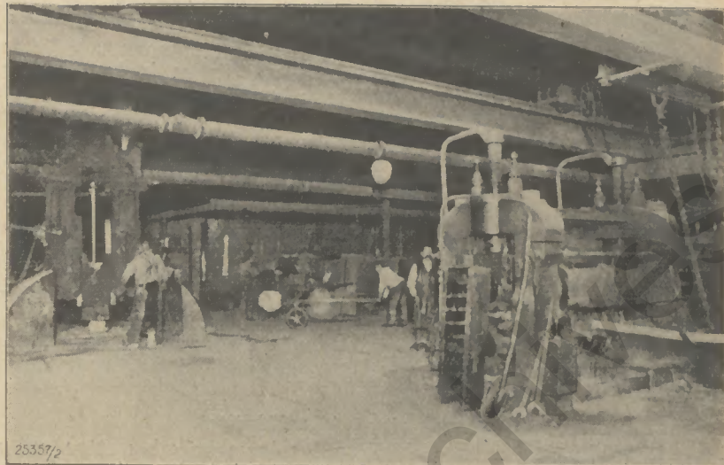
Gesamtansicht des ehemaligen Buddelwerks und Ruppenwalzwerks „Rothte Erde“ in Dortmund
