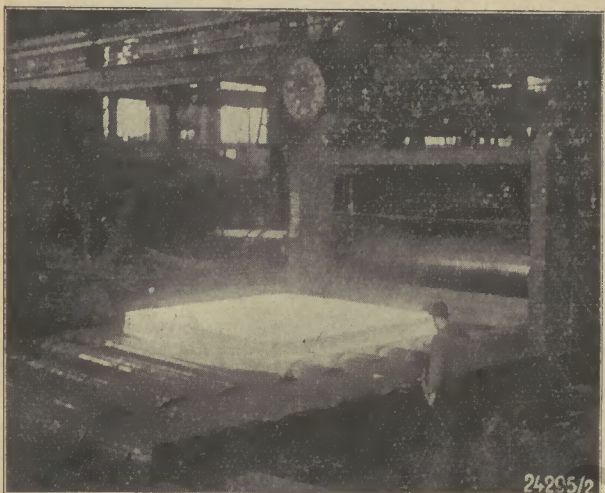
Blechwalzwerk der Stahl- und Walzwerke Thyssen Mülheim, Ruhr
