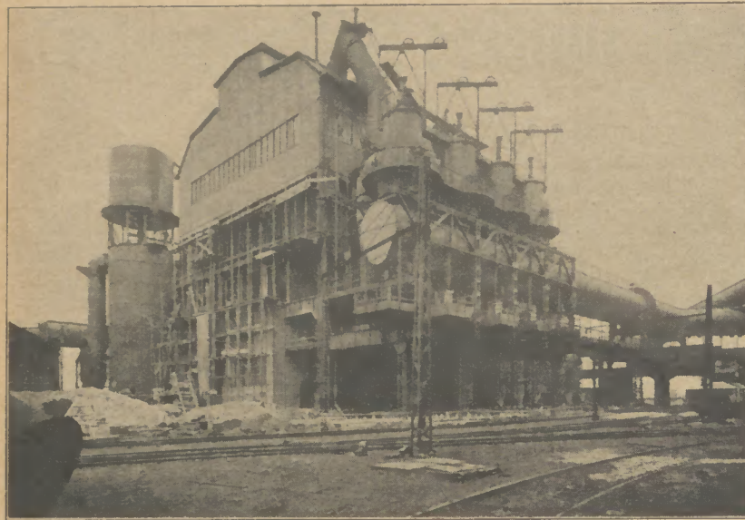
Abb. 10: Trockengasreinigung II, Rohgasseite
