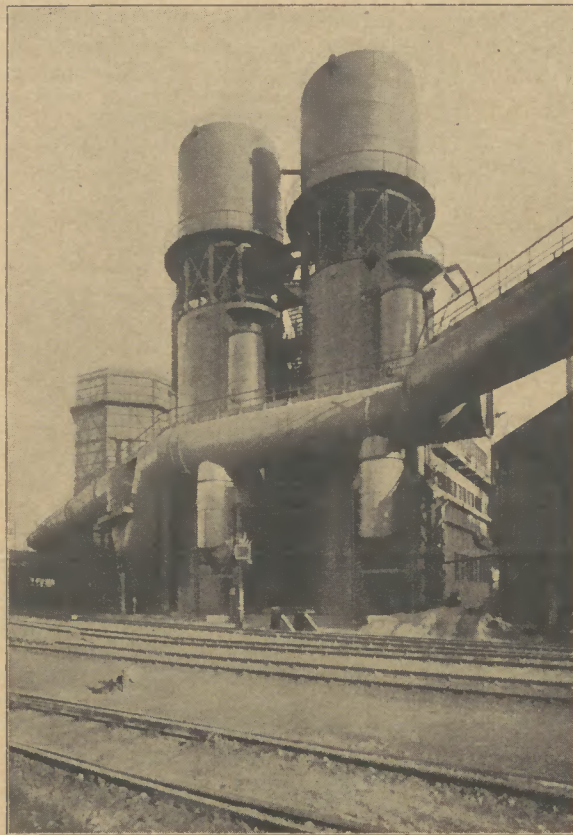
Abb. 12: Nachkühler hinter der Trockengasreinigung II und Reingasleitung, 3 Meter Durchmesser
