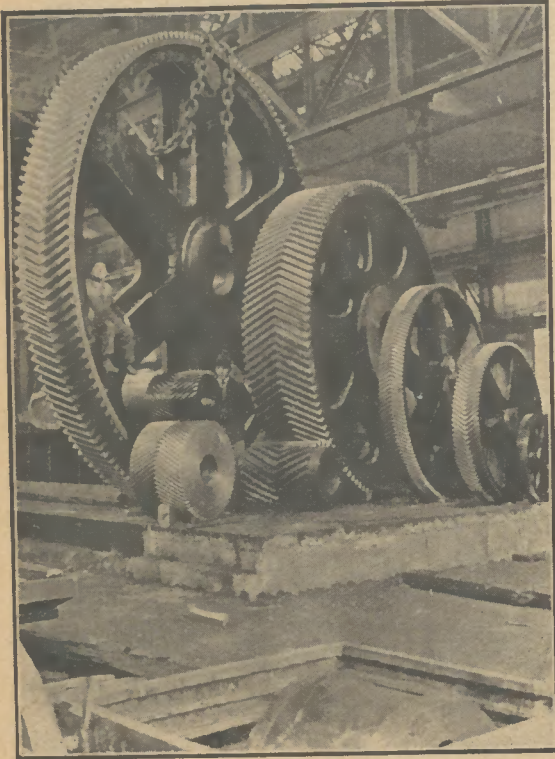
Pfeilzahnräder und Rigel
