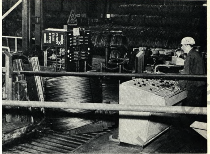
Bild 2: Über einen hydraulischen Kippstuhl werden die Einzelbunde durch einen Abschieber der Presse übergeben.
