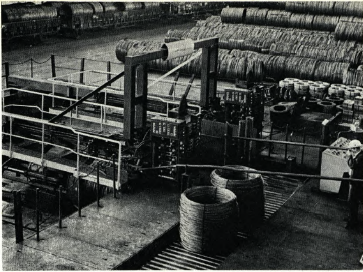
Bild 1: Letzte Station im Produktionsfluß der Drahtstraße IV ist die Großbundpresse.
