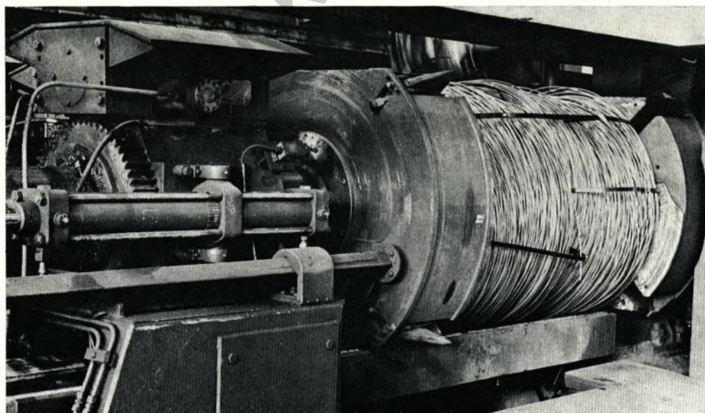
Bild 3: Hier wird das Pressen und Binden der Pakete durchgeführt.
