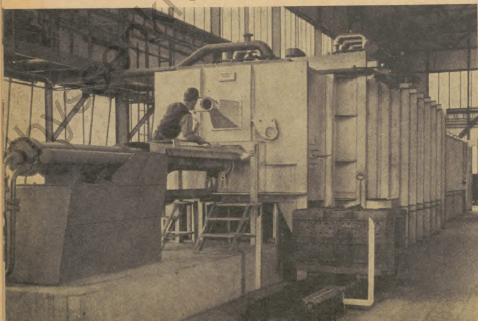
Ofenmann beim Beobachten des eingeschobenen Kastens
