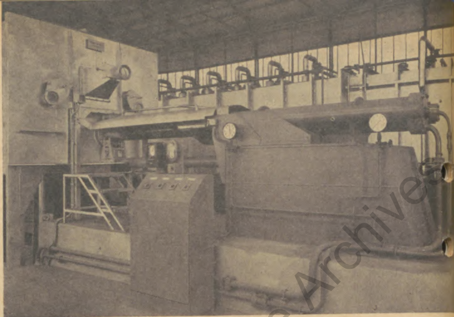
Vorder- ansicht mit Schalt- pult, Block- drücker und Ein- gangs- schleuse
