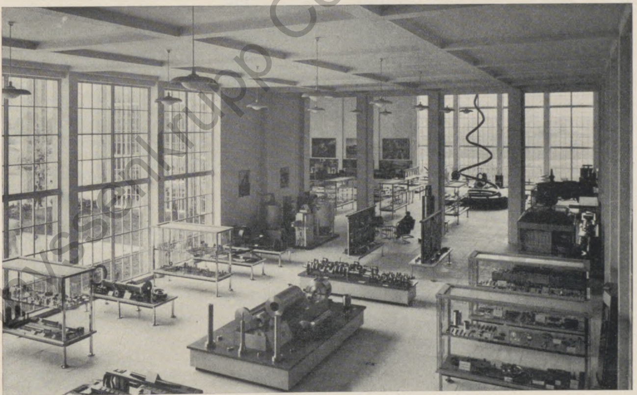
Gesamtansicht der Gemeinschaftsschau „Deutscher Edelstahl“ im deutschen Pavillon; von uns waren ausgestellt: Werkzeuge aus Schnellarbeits- und Werkzeugstahl, Hartmetall Titanit, Werdegang eines Kugellagers, Magnete, Teile aus säure- und hitzebeständigem Stahlguß usw. Belgrad als Messestadt ist das wirtschaftliche Tor zum Balkan.
