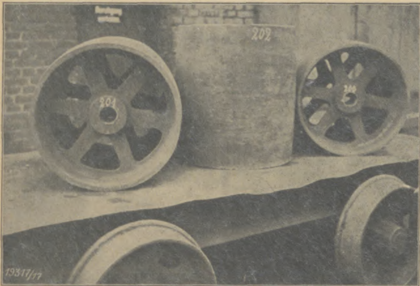
Bild 25: Facharbeit für Lehmformer: Gurttrommel für Transportband (Abguß, gepuht)
