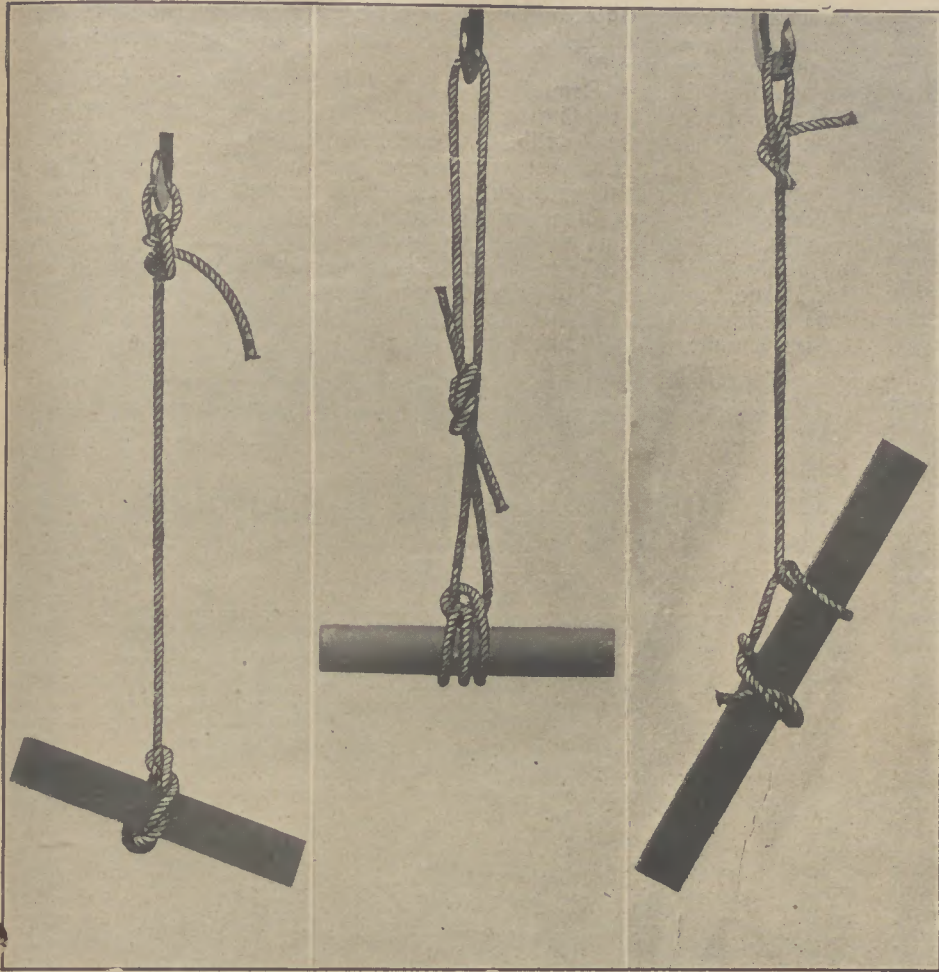
Zimmermannsknoten an der Last, Doppelnknoten am Haken für einfaches Seil (z. B. bei Transport unbelasteter Hölzer.)
