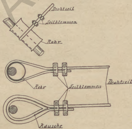
Herstellung von Schlaufen bei Drahtseilen mittels Seilklemmen.
