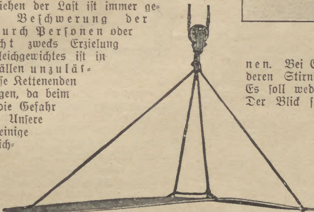
Transport von Platten mittels Anhängen von 4 Ketten.
