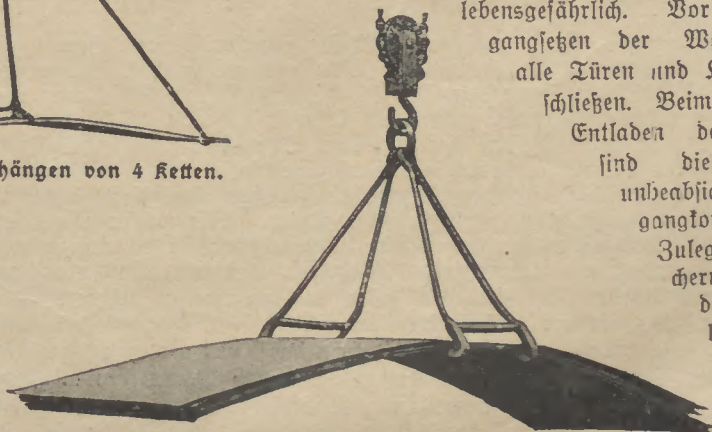
Transport von Platten mittels gekuppelter Traghaken.
