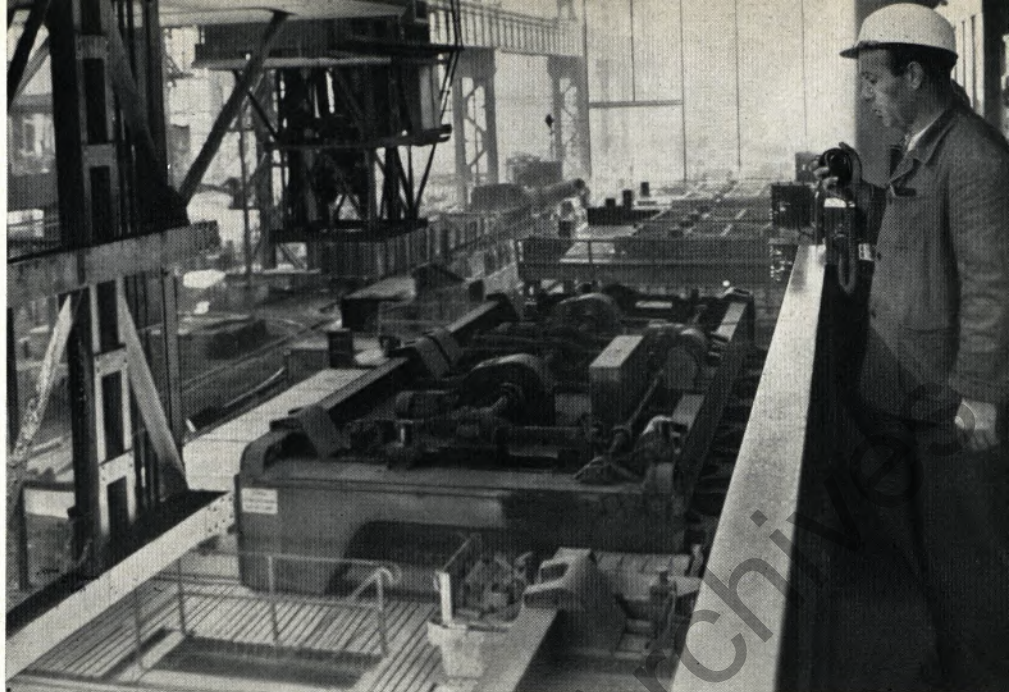
1. Tiefofenmann Ewald Lechtermann dirigiert durch Sprechfunk mit dem Kranführer den Tiefofeneinsatz. Im Bild links erkennt man die Kranbahn und den Kran, in der Bildmitte befinden sich die Tiefofen.
