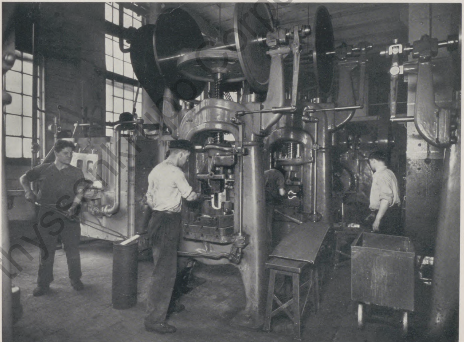
Warmpressen der Magnete
