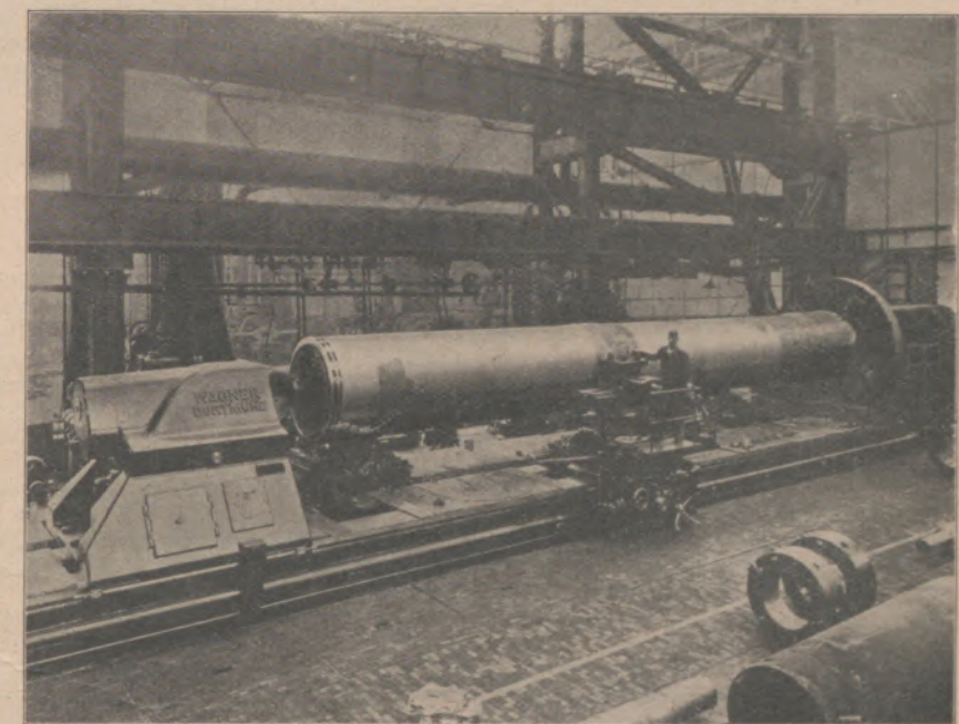
Bild 5: Die fertig geschmiedete Trommel von 13 Meter Länge und 1,55 Meter Durchmesser auf der Drehbank in der Preßwerk-Werkstatt
