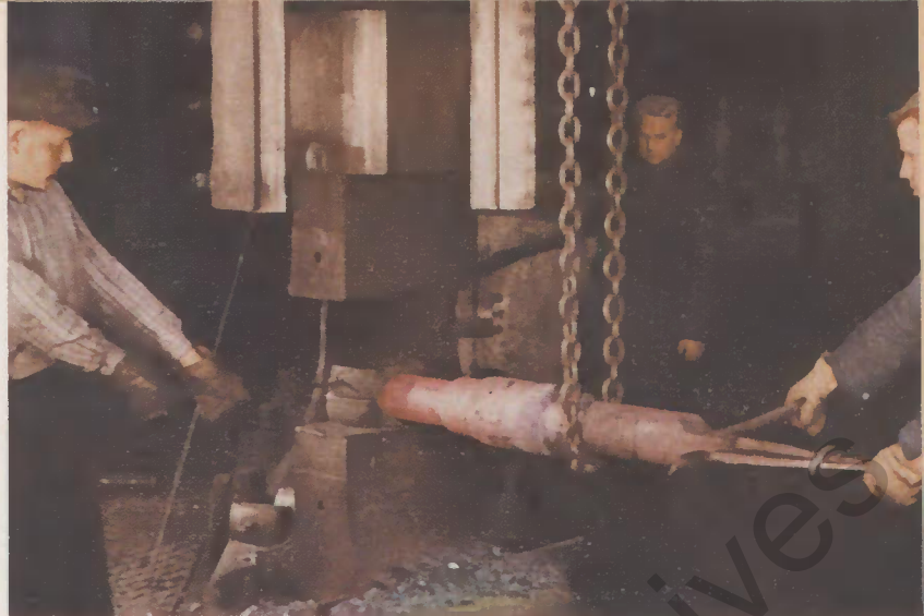
Vorschmieden einer Achse. Von links nach rechts: H. Lederhose, H. Desel, J. Schäfer.
