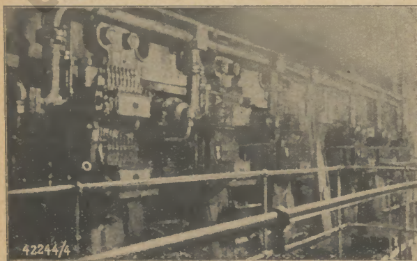
Manöverierstand und Hauptmaschine des Motor- schiffes „Duisburg“
