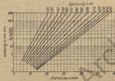
Belichtungsschaubild für Röntgenaufnahmen
