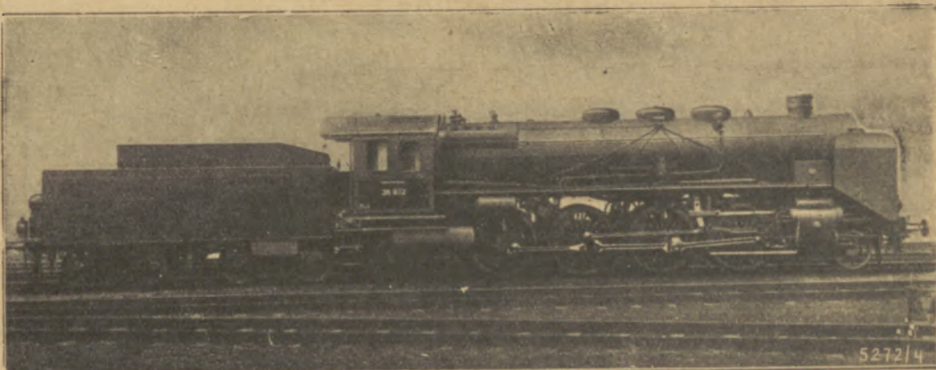
Dreizylinder-Heißdampf-Personenzug-Lokomotive der Firma Fried. Krupp A.-G. 14 atü, Dienstgewicht 111 t, Leergewicht 100 t, Geschw. bis 110 km i. d. Std., Leistung 1000 PS.
