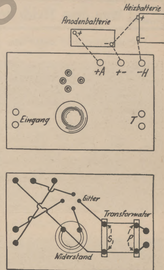
Abb. 2: Bauzeichnung des Verstärkers.
