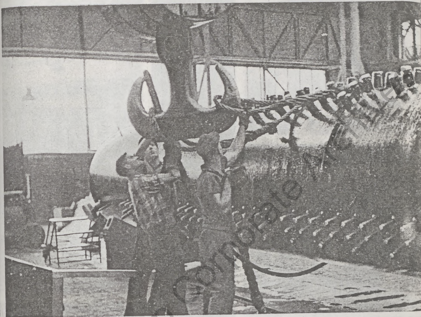
Der Riesenkesseltrommel wird eine Krawatte aus Hanf um den Hals gelegt.
