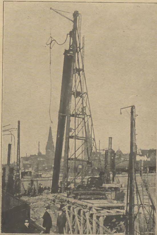
Hochgezogene Bohle kurz vor dem Rammen.
