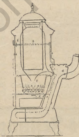
Amerikanischer Dauerbrenner
