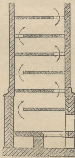
Kachelöfen
