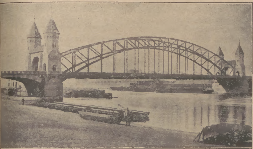
Eisenbahnbrücke über die Weser bei Nienburg. Halbparabelträger mit Zwischensystem.
