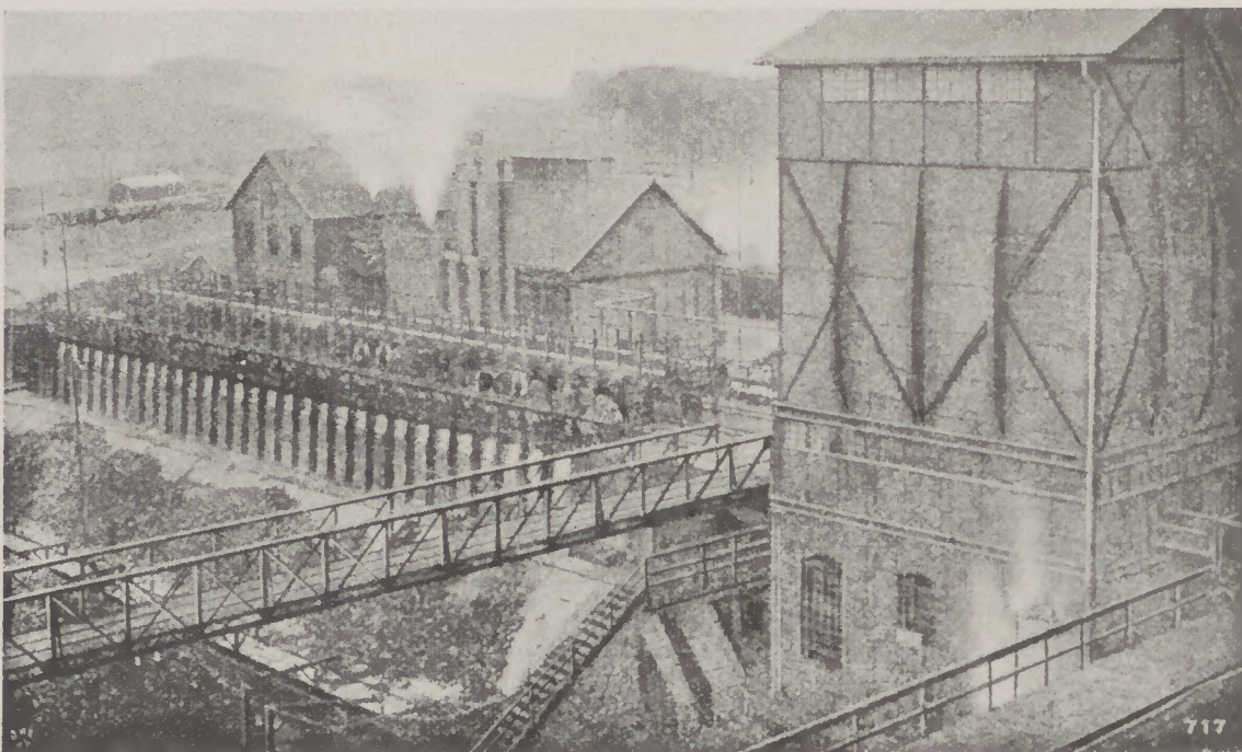
Kokerei (30 Öfen) mit Gewinnung der Nebenprodukte „System Brund“ auf dem Eisen- und Stahlwerk Hoesch, Dortmund. Erbaut 1898
