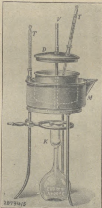
Abb. 3: Zähigkeitsmesser für Öle konstruiert von Engler.
